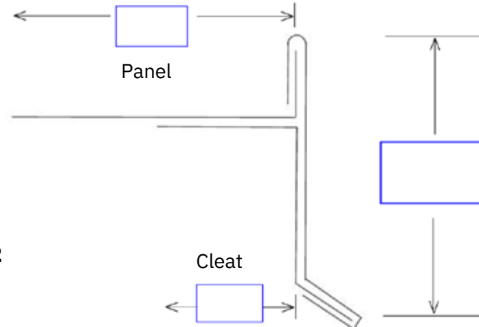
Alternate Rake Edge Detail #2
